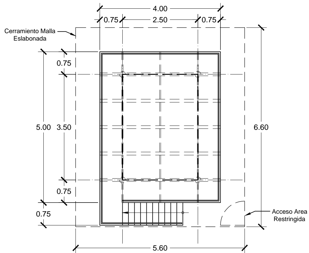
PLANTA N. +2.20
